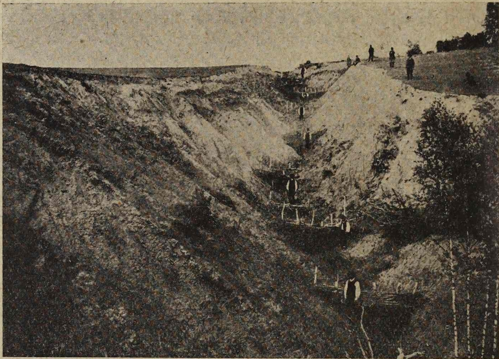
161. ábra. Rőzsegátkötések Erdélyben a székelyföldi ministeri kirendeltség legelőjavítási munkálatainál.
