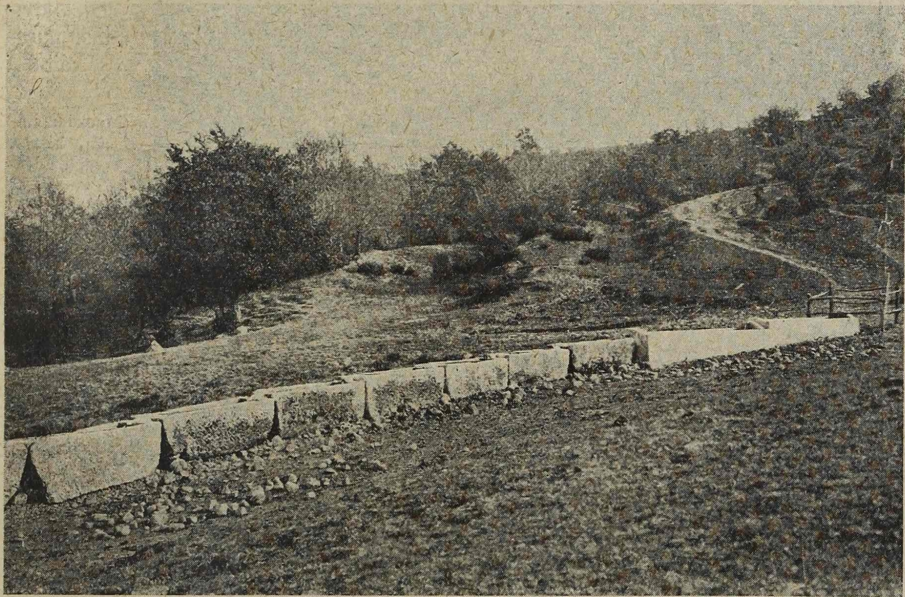
283. ábra. Beton- és kővályuk, földalatti csővezetékekkel Udvarhely megyében. (Székelyföldi miniszteri kirendeltség legelőjavítási munkái.) (Munkám számára készült eredeti föl vétel.)
