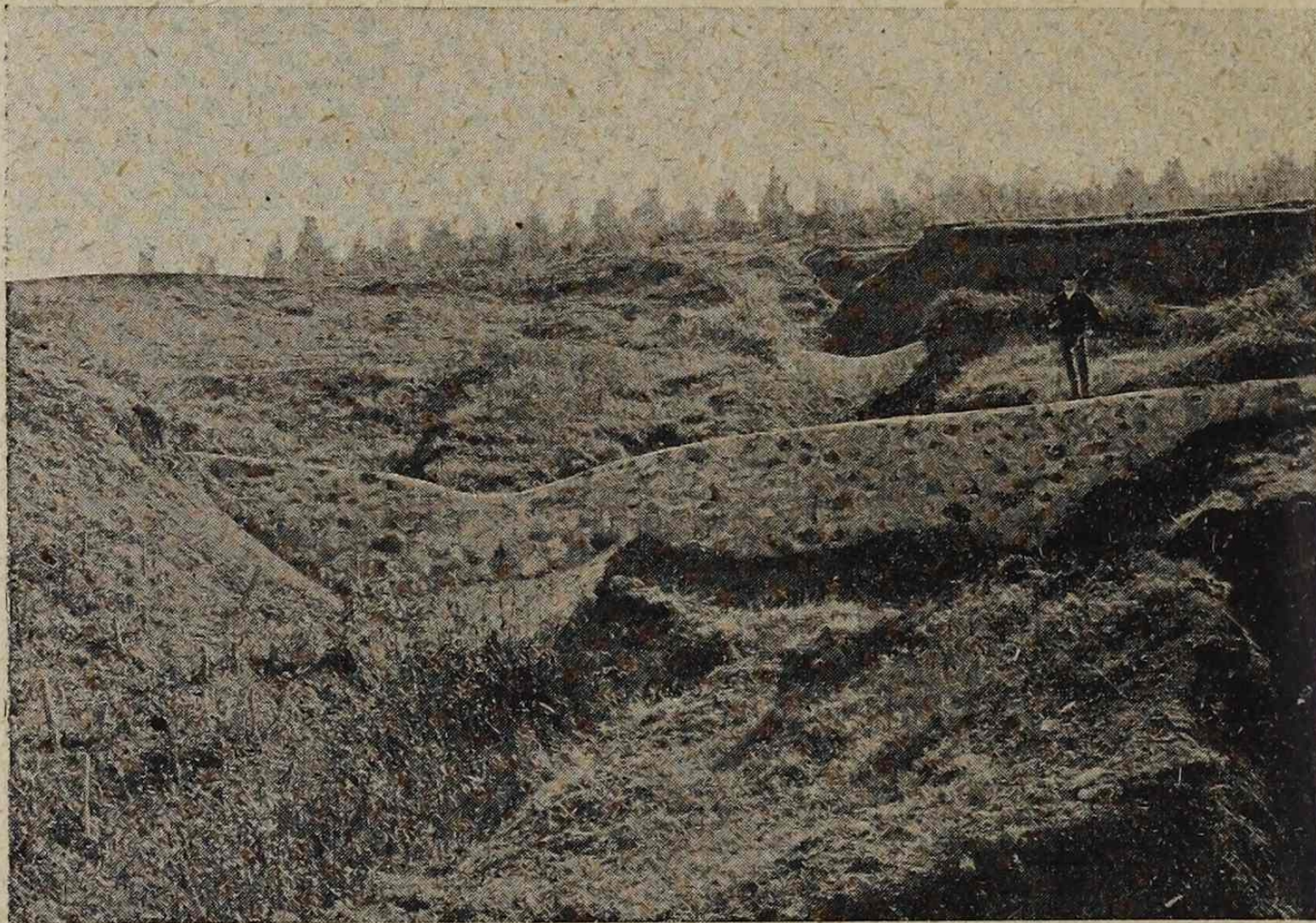
159. ábra. Vízmosásoktól összeszaggatott és csúszó („suvadó“) talaj megkötése cementberakott terméskögáttal Udvarhely megyében, a miniszteri kirendeltség legelőjavítási munkálatainál.
