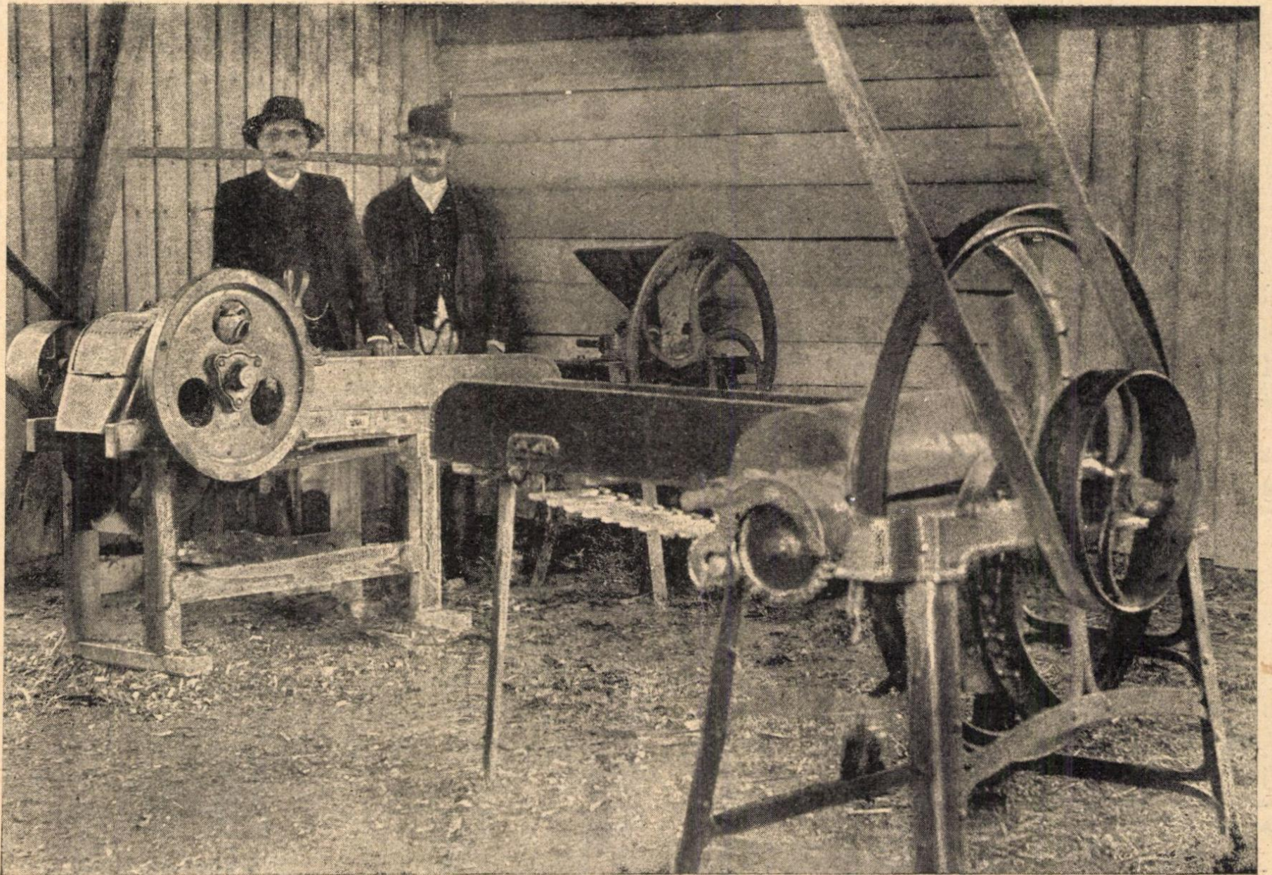
41. ábra. A szecskavágó csarnok belső képe.
