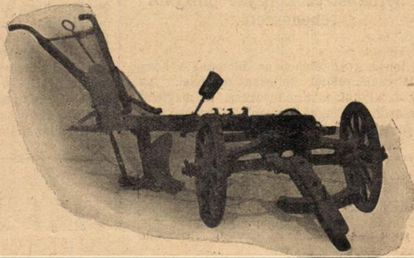
239. ábra. Ikerváltó eke szántásra váltva, jobbfelé vető ekeállással.
