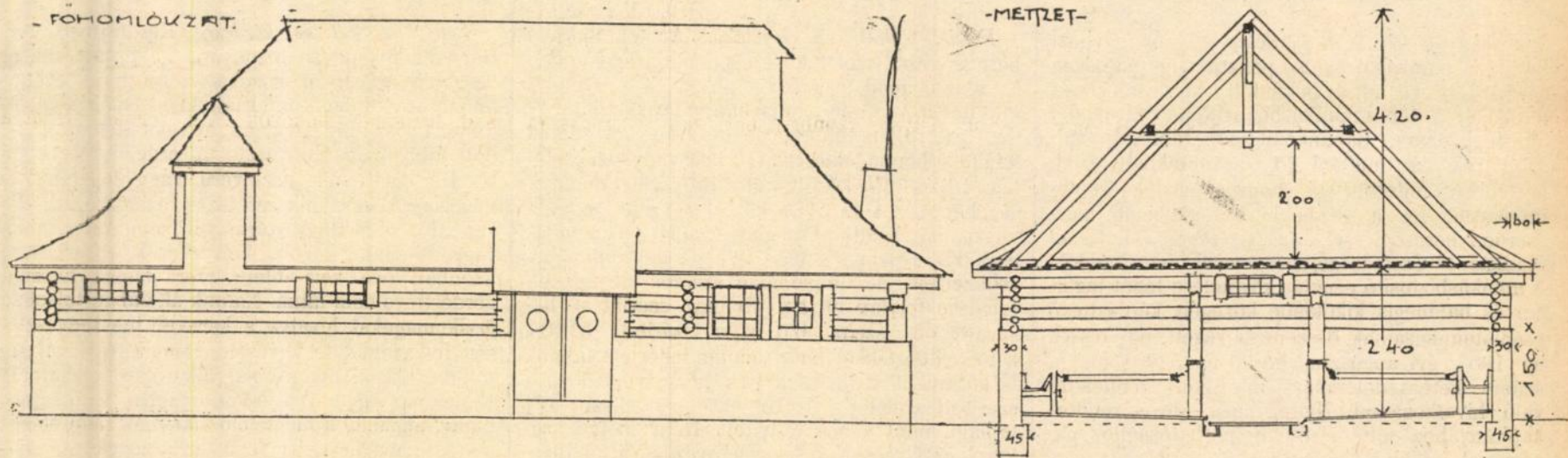
182. ábra. Székely falusi bikaistálló keresztmetszete és főhomlokzata. (Wiegand-féle székely stilizálással.)
