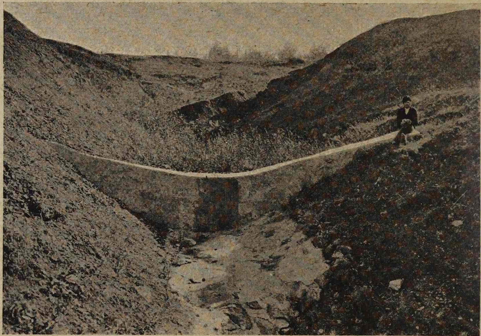
166. ábra. Betonból készült gát és cementtel kivakolt árokfenék egyik udvarhelymegyei legelőn. Munkám részére készült eredeti fölvétel.
